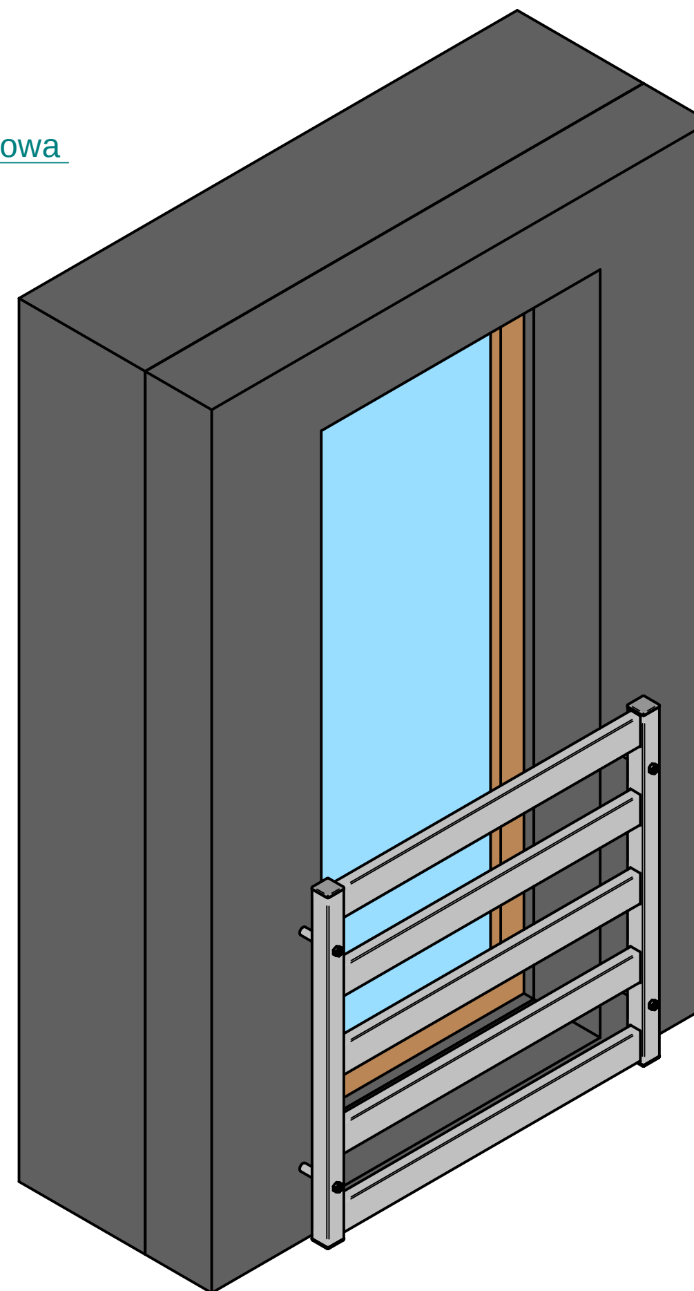
BALUSTRADA 80x30 Montaż do sciany z dystansem
